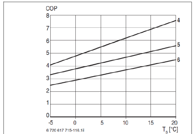
Bild 41 Leistungszahl STE 130-1
