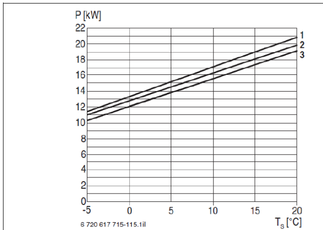
Bild 40 Leistungsdiagramm STE 130-1
