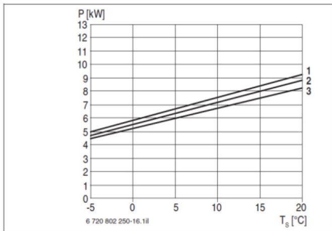
Bild 34 Leistungsdigramm STE 60-1
