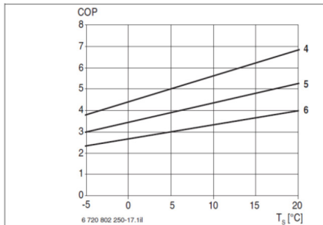
Bild 35 Leistungszahl STE 60-1
