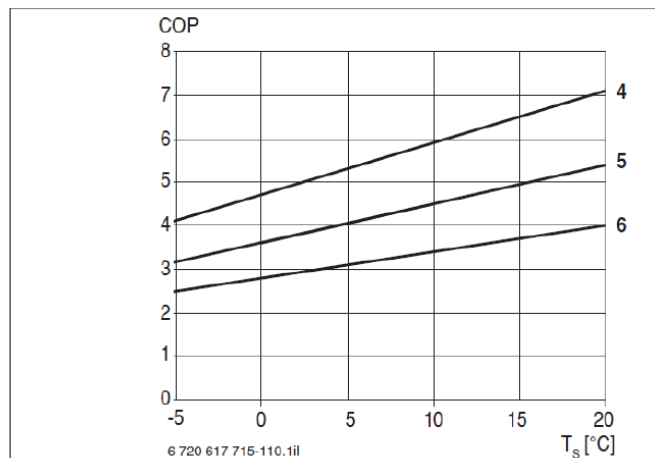
Bild 37 Leistungszahl STE 80-1
