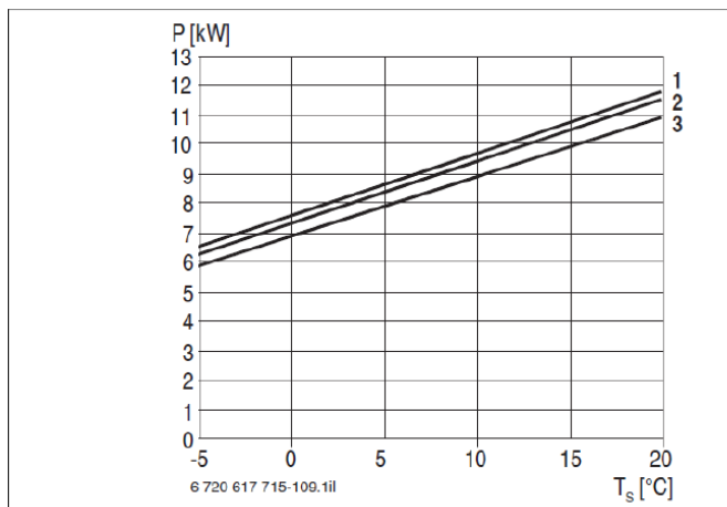
Bild 36 Leistungsdiagramm STE 80-1
